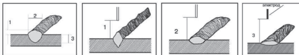
Рис.5 1 - высота направленного металла, 2 - ширина наплавленного металла, 3 - глубина проникновения Напряжение дуги малое Напряжение дуги среднее Напряжение дуги высокое 1 - малая длина дуги, 2 - средняя длина дуги, 3 - большая длина дуги Рис.6
